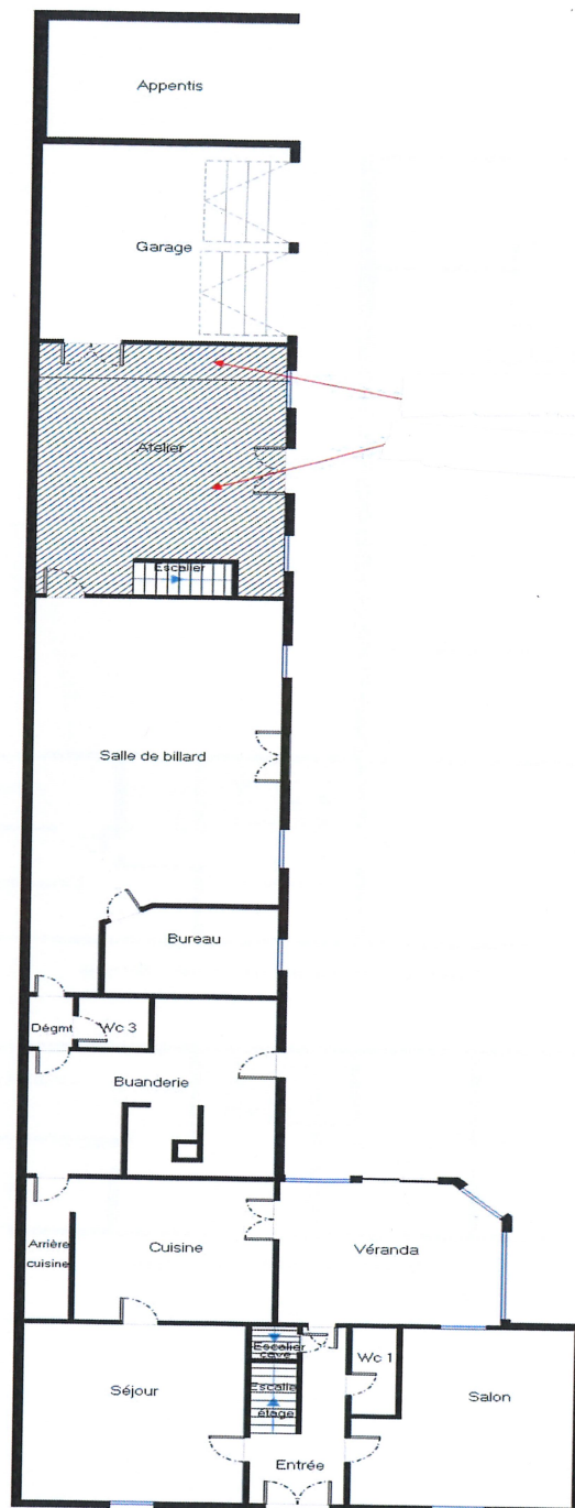
Plan de masse rez-de-chaussée
